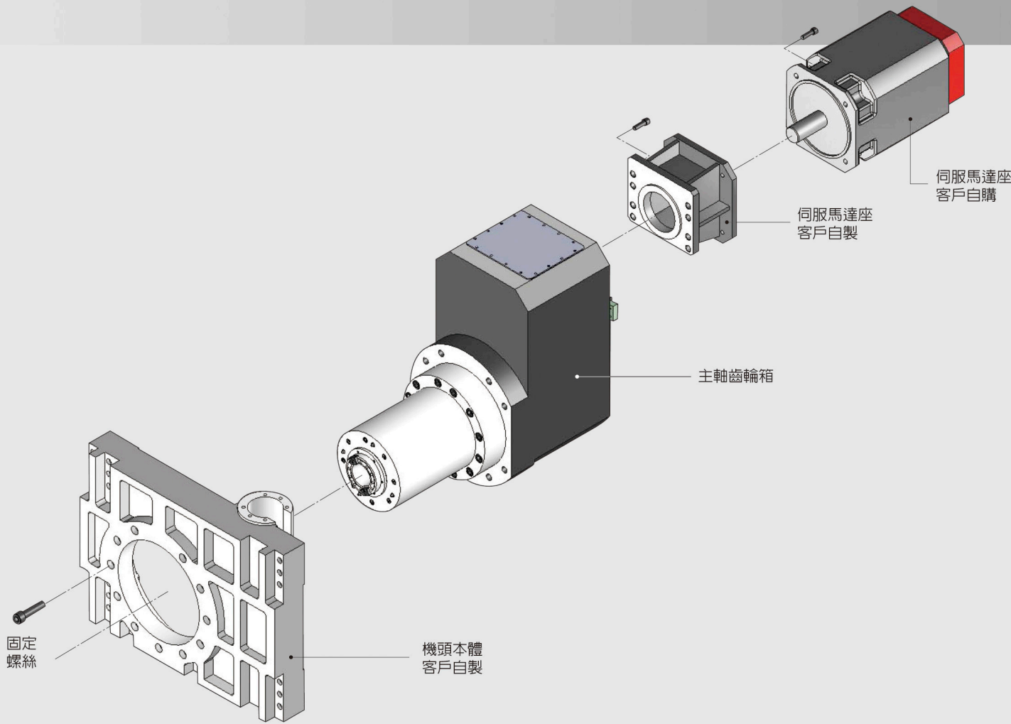
》臥式機頭組裝圖
